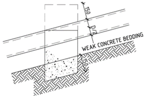
LONGITUDINAL SECTION
