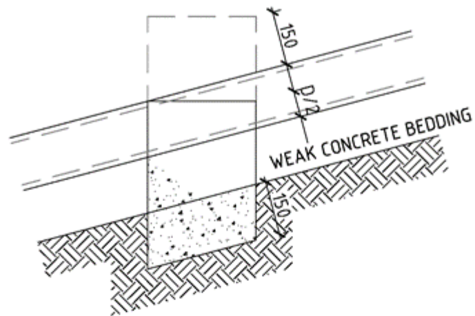
LONGITUDINAL SECTION
